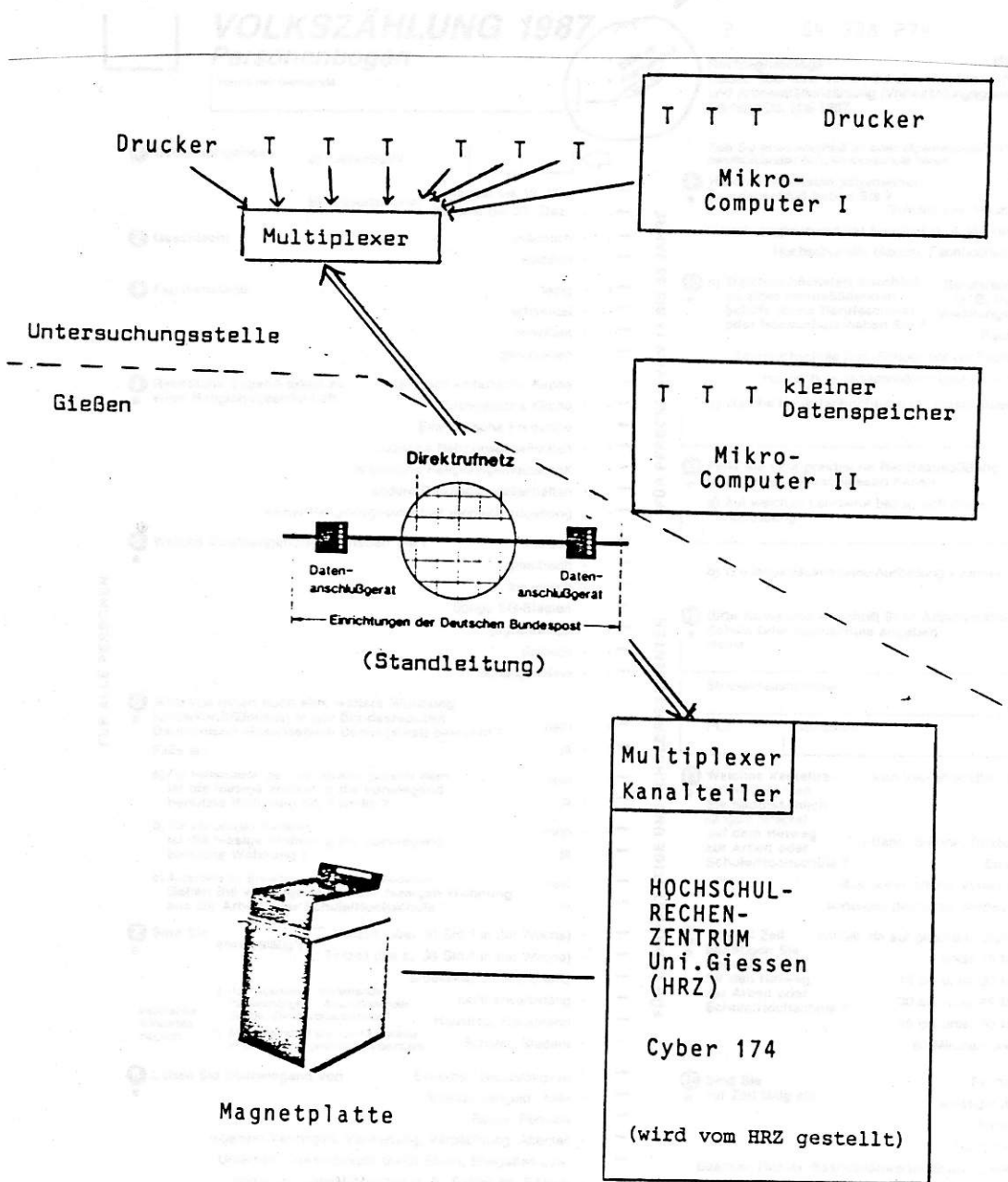
Abb.612 Plan für das Gesamt-System der elektronischen Daten-Verarbeitung für eine ernährungsepidemiologische Studie im Jahr 1983*
