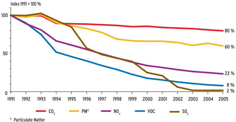
Spezifische Emissionen Pkw (Emissionen Pkw/Verkehrsleistung Pkw)
