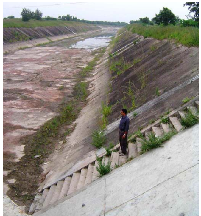
Falsch geplanter Bewässerungskanal in der Provinz Andhra Pradesh in Indien © WWF
