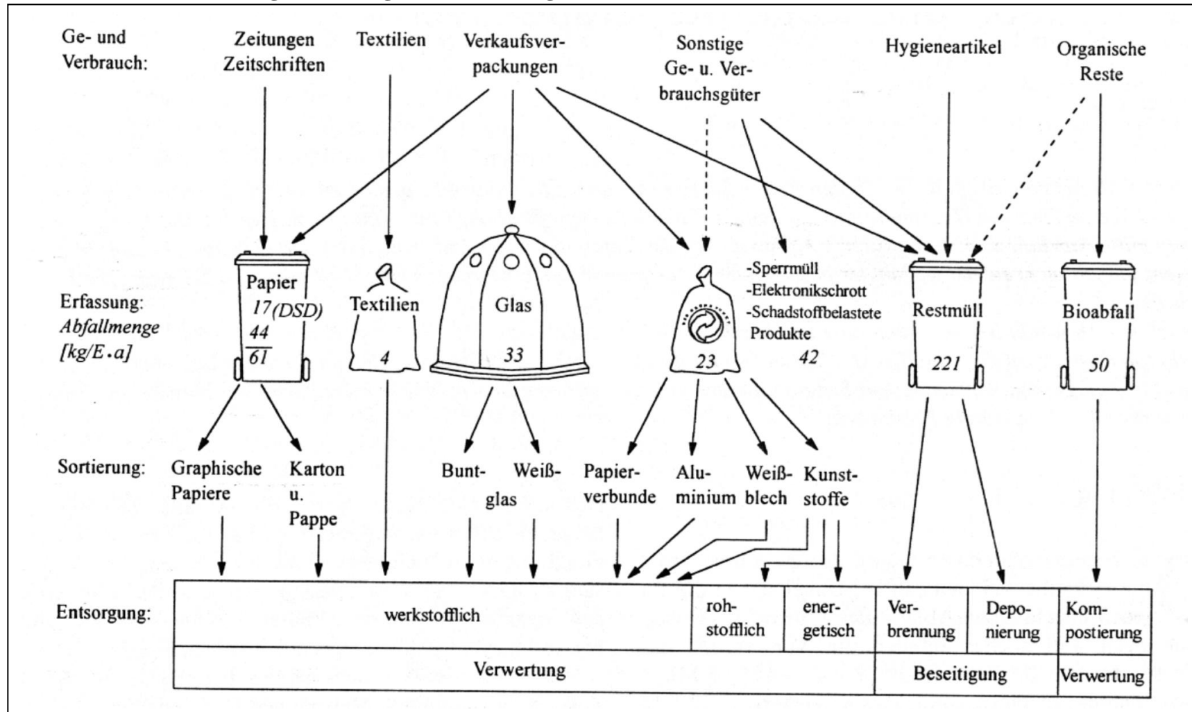
Abb. 4.8: Aktuelle Erfassung, Sortierung und Verwertung von Hausmüllbestandteilen
